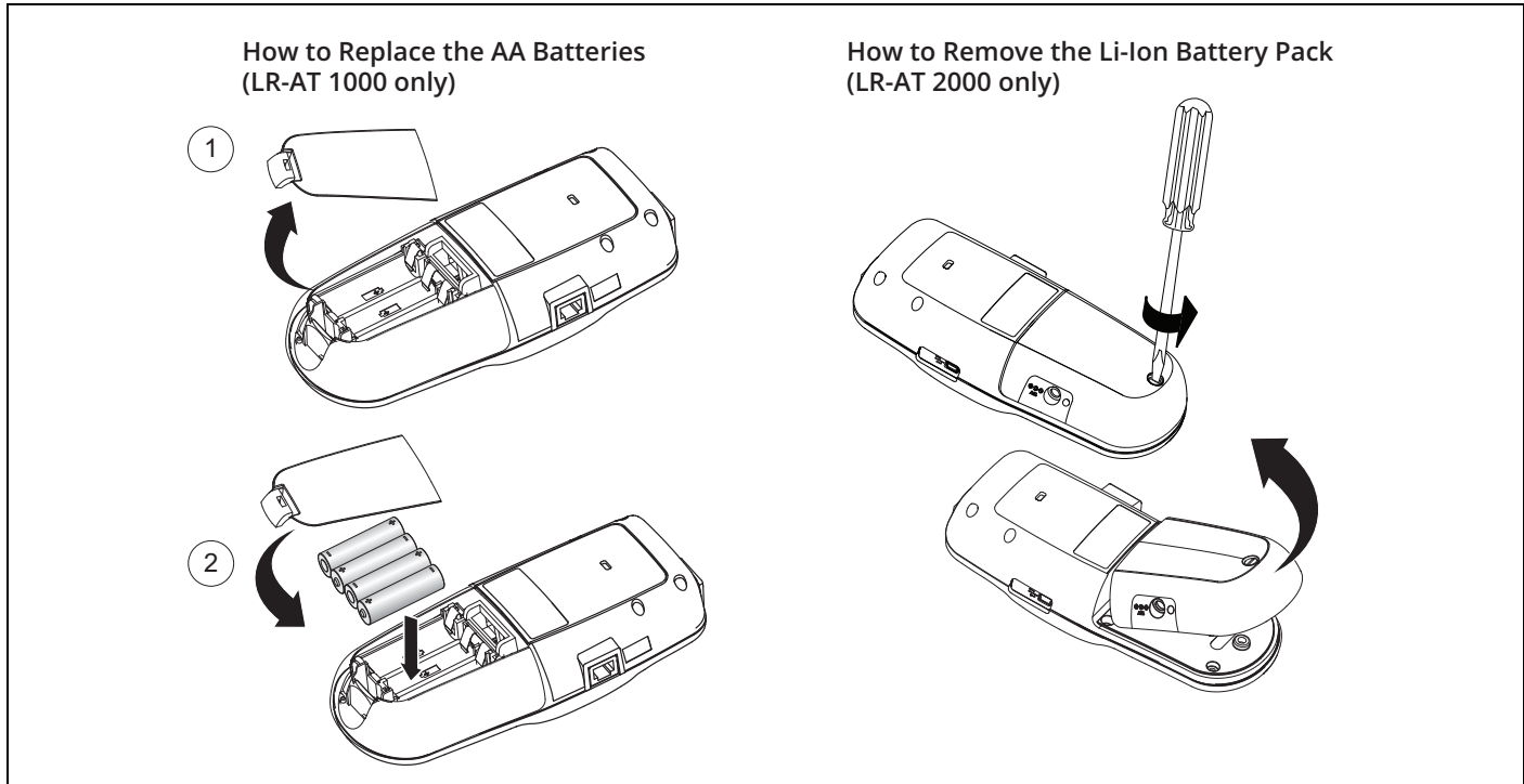
Рис.2. Извлечение или замена аккумуляторов
